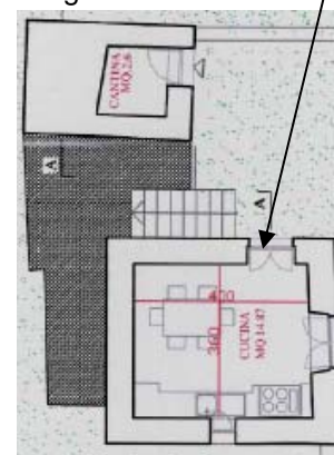
Erdgeschoss
