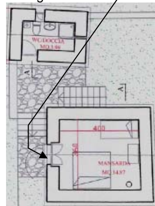
Obergeschoss
